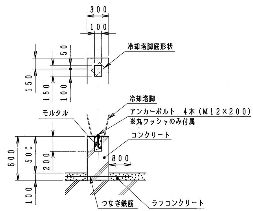
基礎参考図
