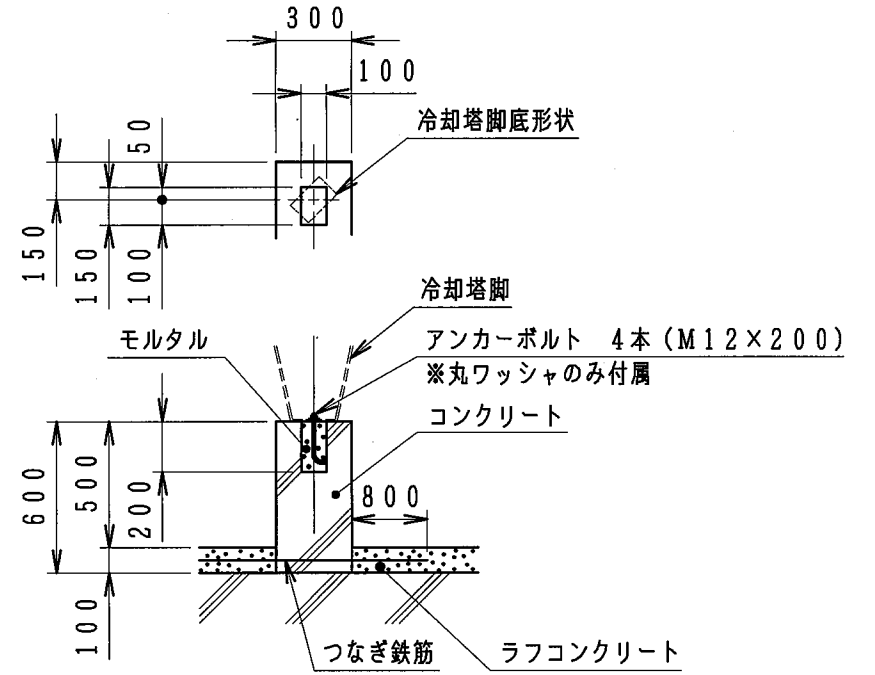
基礎参考図
