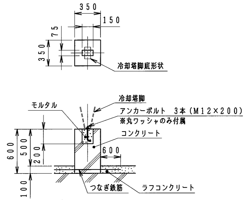
基礎参考図
